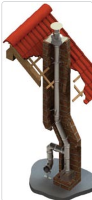
Béléscső rendszer (nem túlnyomásos)
