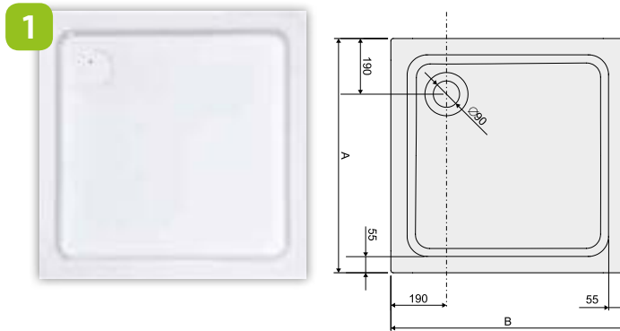
A fotón látható: B/FREE 90x90x5 bi zuhanytálca, előlappal szerelve
