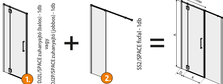
A fotón látható: DJ2L/SPACE 120 sb W0 ajtó (átlátszó üveggel) + SS2/SPACE 50 sb W0 kiegészítő fal A fotón balos kivitel látható! Az SS2 toldó falban nincs jobbos vagy balos kivitel. A toldó fal átfordítható!
