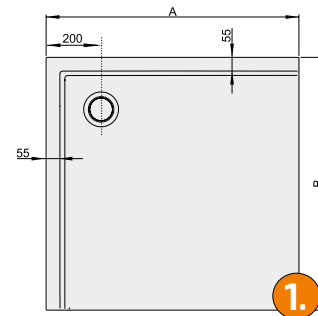
A fotón látható: B-M/SPACE 90x160x1,5 bi zuhanytálca (fölnézet)
