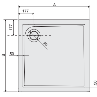
Bza/PR négyzetes sicaljű tálca
