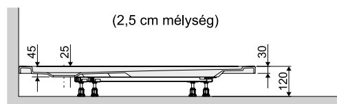
A fotón látható: BP/FREE 90x90x2,5 bi zuhanytálca
