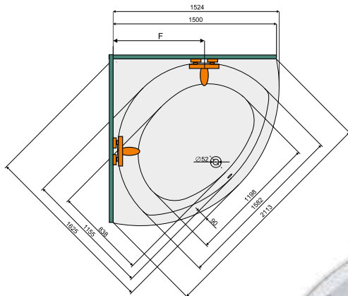
A fotón látható: WS/PR 150x150 bi fürdőkád, hidegburkolattal burkolva
