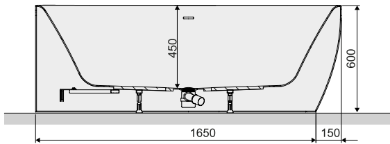
A fotón látható: WAPse-kpl-mb/LUXO 80x180bi fürdőkád, gyárilag egybeöntve (jobbos)
