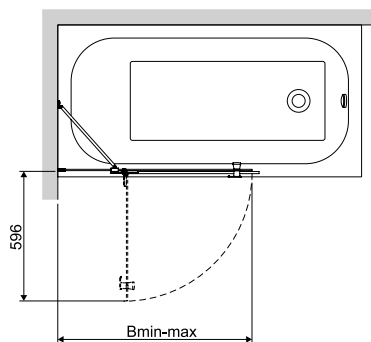
Kivitel: rövid fix elem + nyíló rész (nyílórész kifelé nyitható!)
