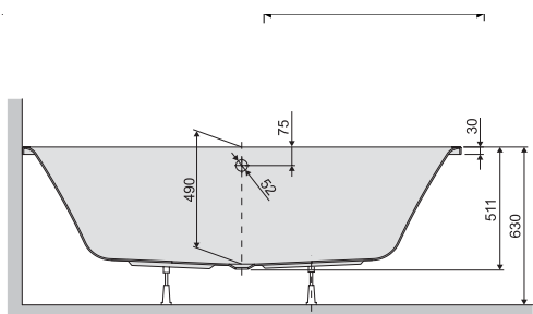
A fotón látható: WP/LUXO 80x180bi fürdőkád
