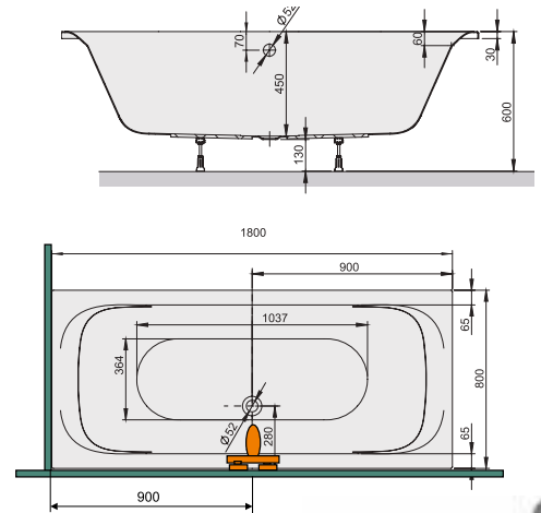
A fotón látható: WPdo/BASIC típus (középlefolyós)
