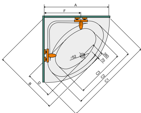
A fotón látható: WS/FREE bi-fürdőkád, előlappal burkolva
