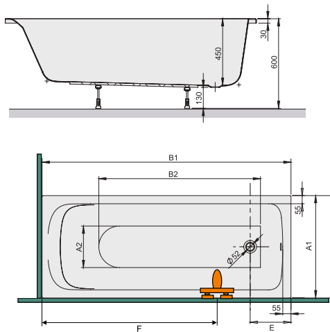
A fotón látható: WP/BASIC típus (véglefolyós)
