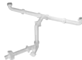
BAZOOKA SPACE helytakarékos szifon dupla mosdókhoz 1"1/4 32x230 2920CP32B0 3.490,-
